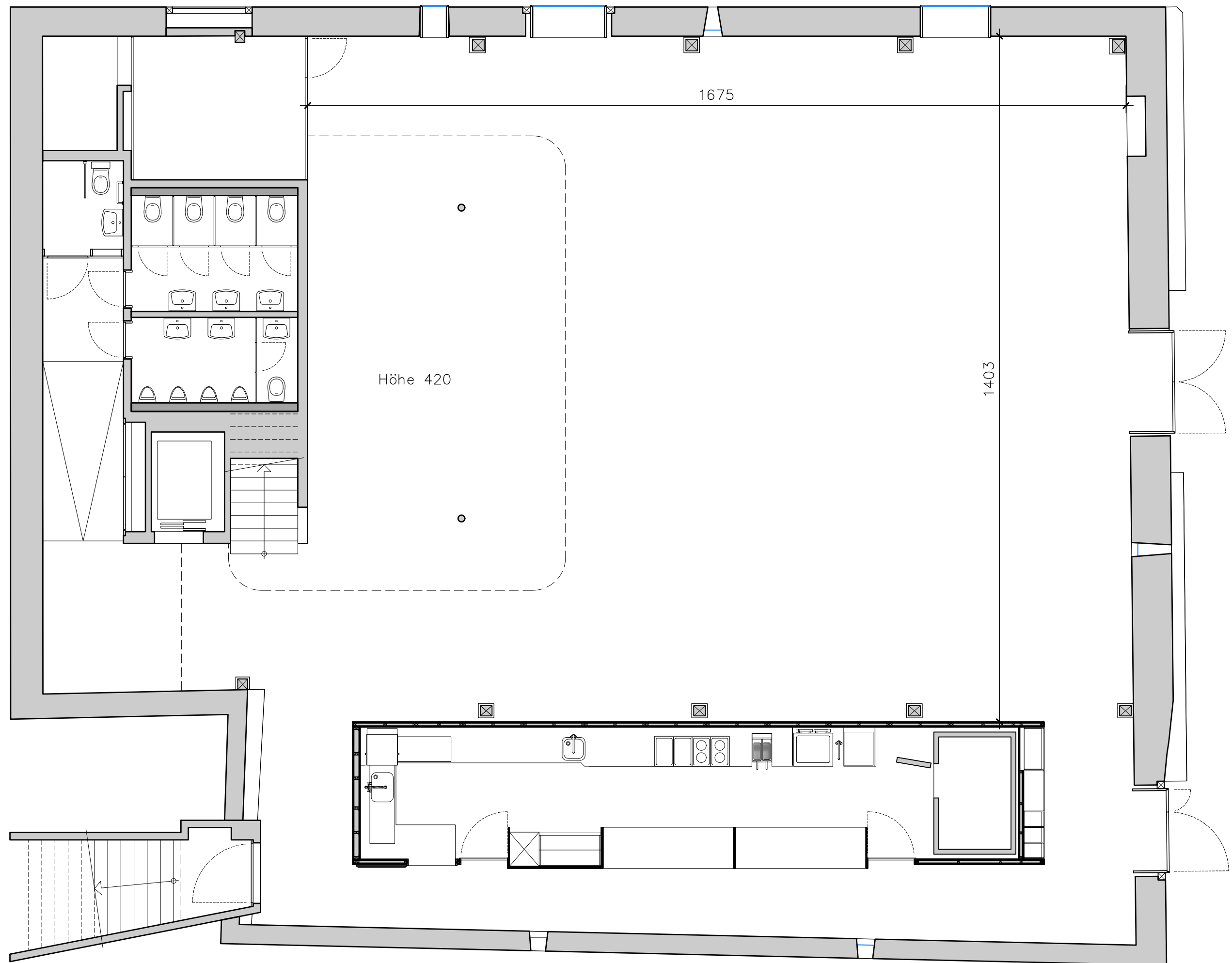
Trotte Villigen - Festsaal Erdgeschoss
